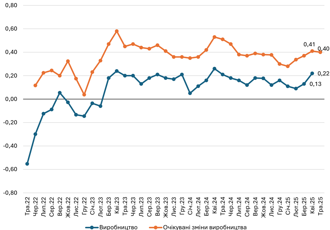
Виробництво, балансові показники
